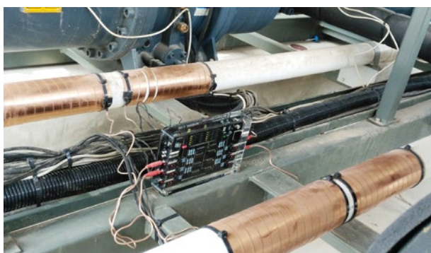
Vulcan S100 a été installé sur le dispositif principal de climatisation
