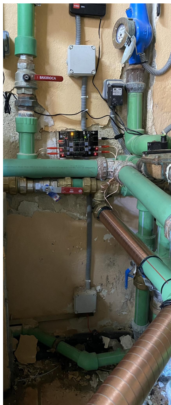
Vulcan S50 sur le tuyau d'eau froide de Ø 63 mm
